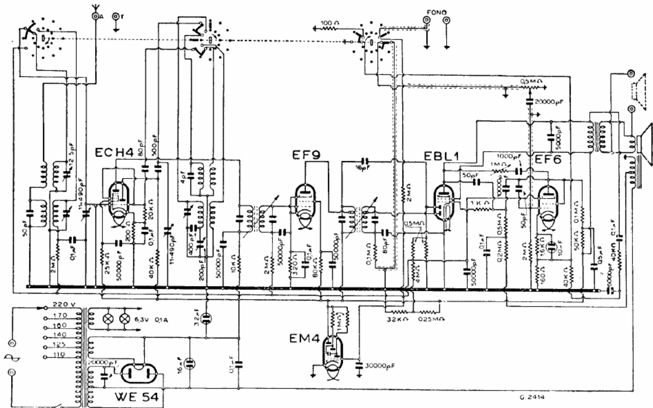
Lo schema elettrico del mod. 466
